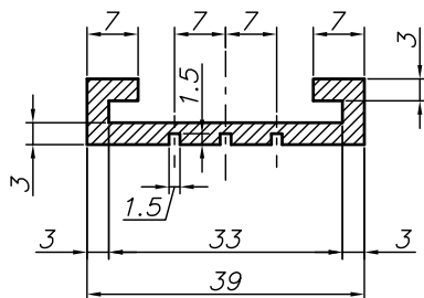
防振ゴム断面
