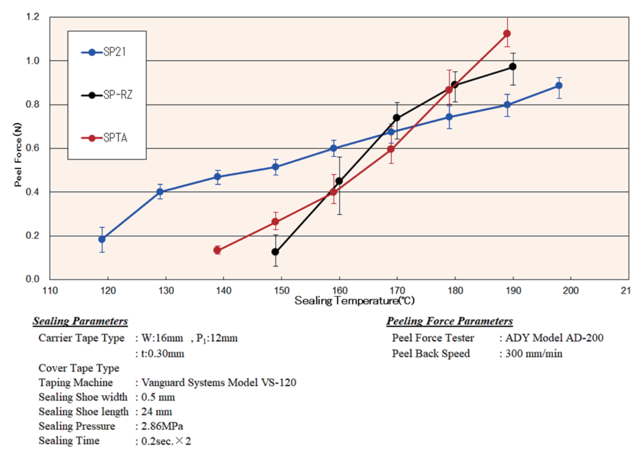
シール温度性 測定結果(PS導電タイプ*SP21)
