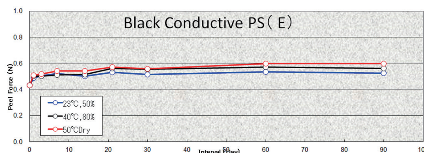
経時変化 測定結果(PS導電タイプ*SP21)
