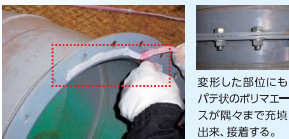
U字ピット内本管で自己融着テープ使用不可の狭小現場で採用
