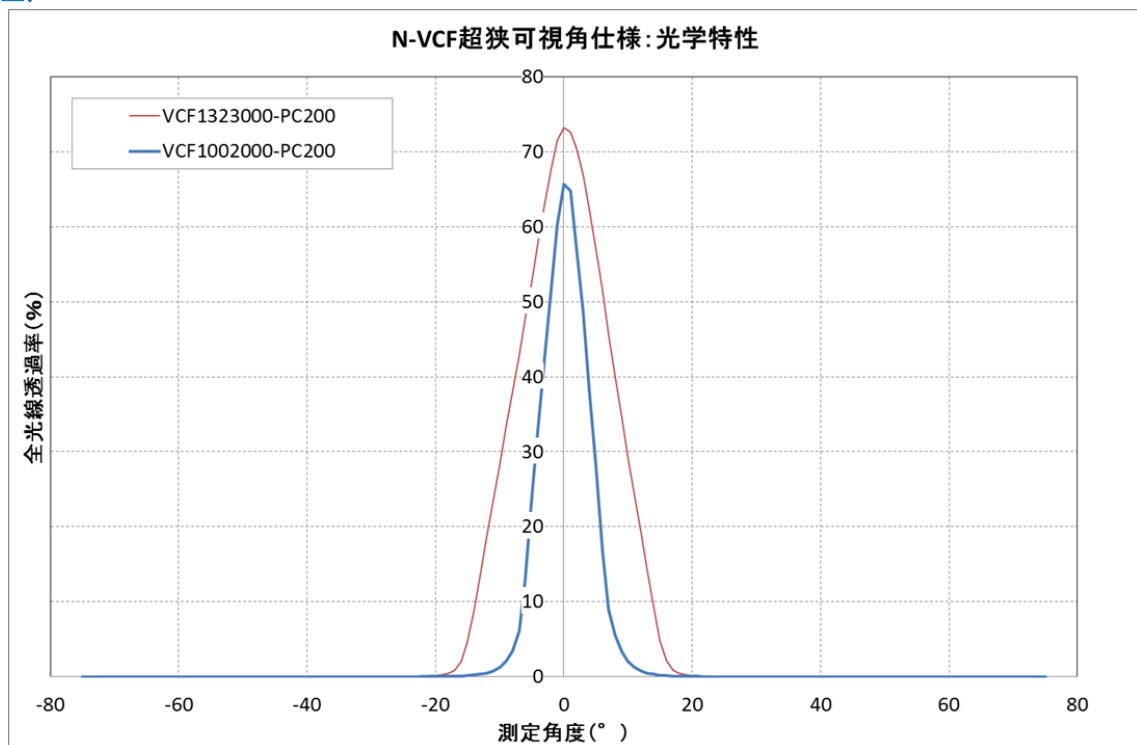
N(Narrow)-VCF TYPE : Single louver : N-VCF 1323000-PC200
