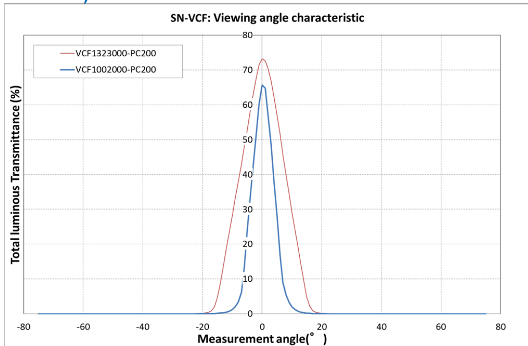
N(Narrow)-VCF TYPE : Single louver : N-VCF 1323000-PC200
